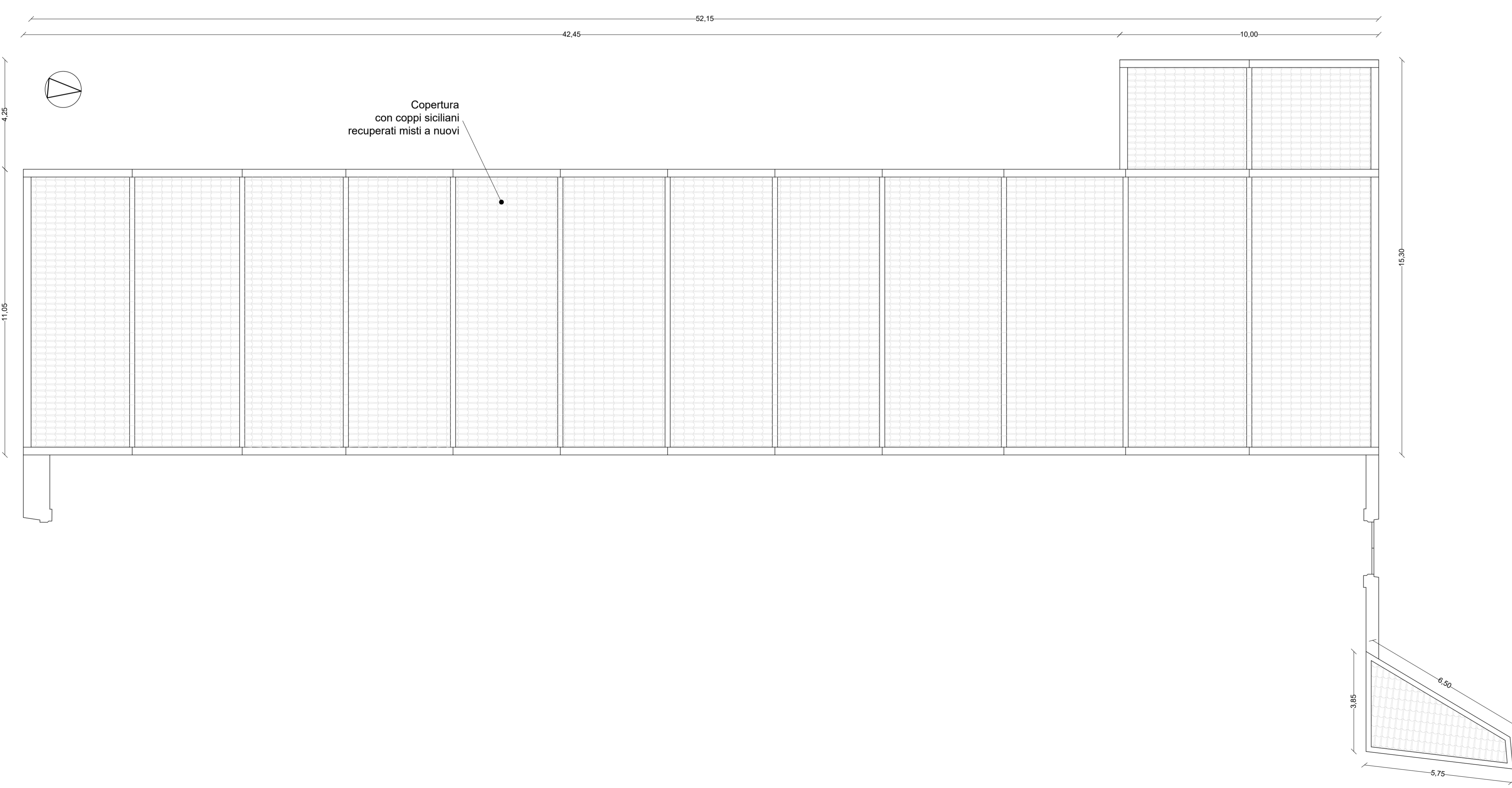
PIANTA COPERTURA
